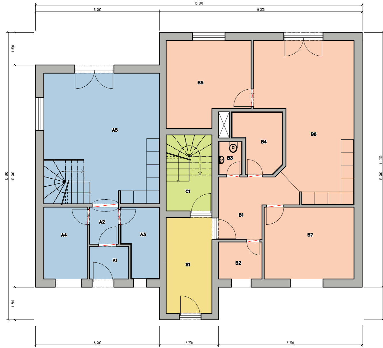
PŮDORYS 1NP - 1:100
