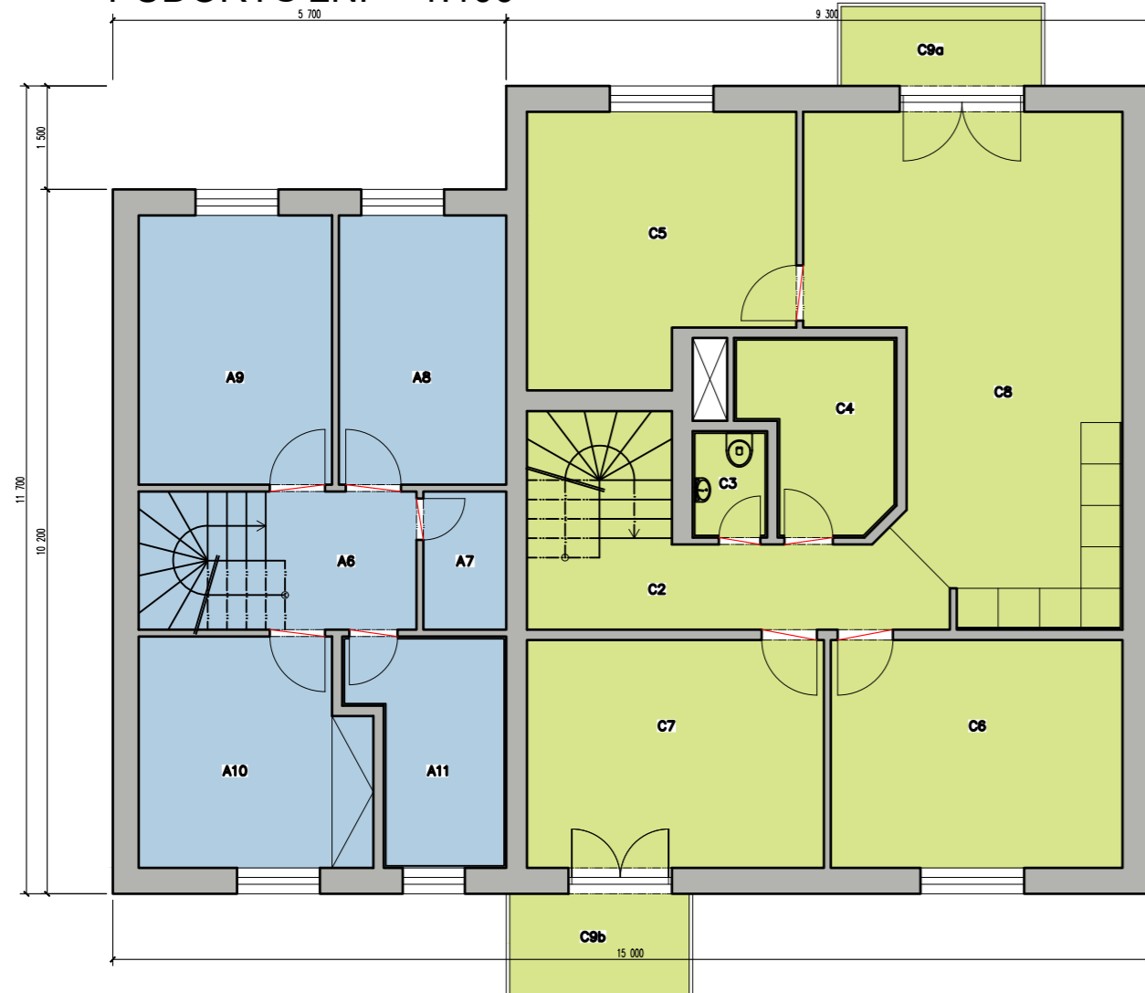
PŮDORYS 2NP - 1:100
