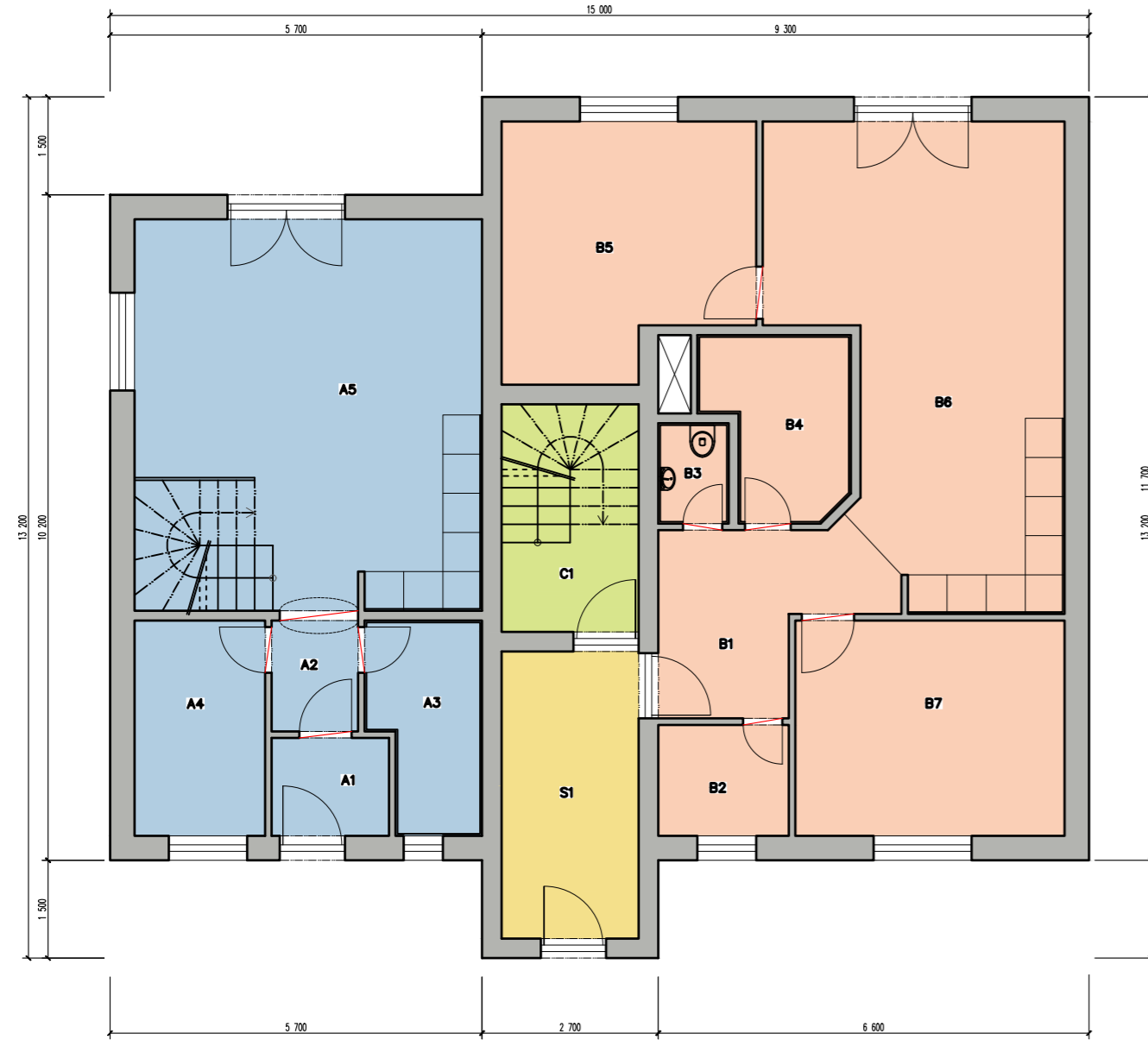
PŮDORYS 1NP - 1:100
