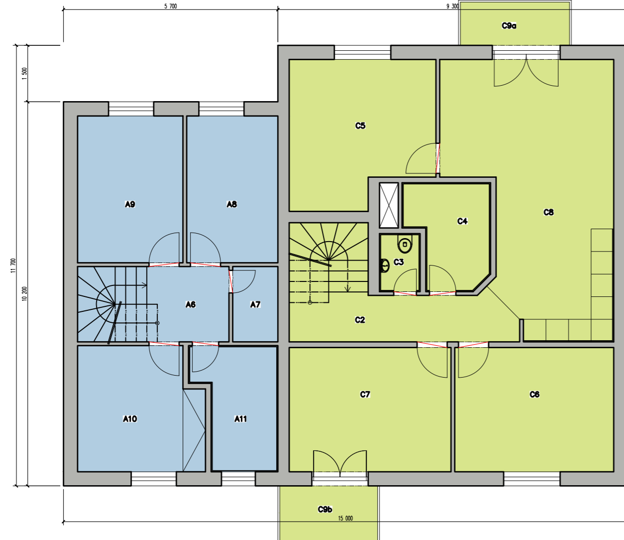
PŮDORYS 2NP - 1:100
