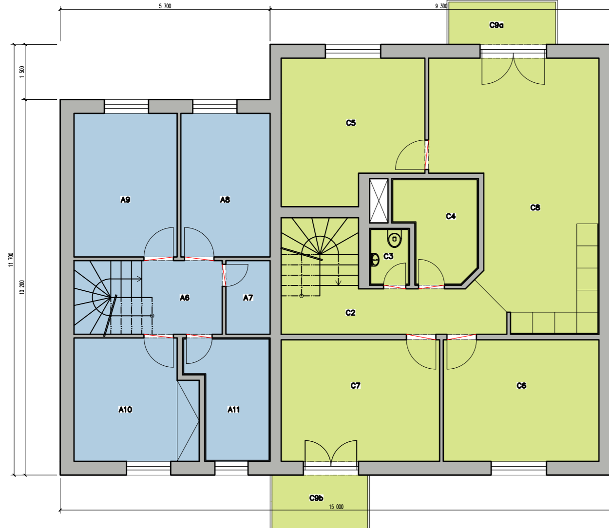
PŮDORYS 2NP - 1:100
